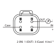
Deutsch DT04-4P
