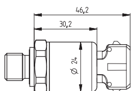
AMP JPT
